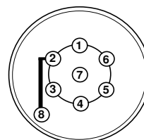
Pod³czenie przewodów w gnie¿dzie 7-biegunowym
