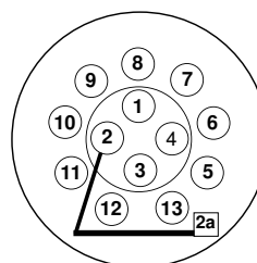
Pod³czenie przewodów w gnie¿dzie 13-biegunowym
