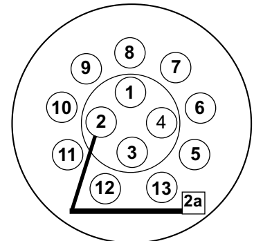
Kontaktbelegung 13 pol der Steckdose
