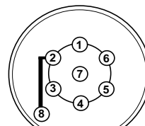
Podłączenie przewodów w gnieździe 7-biegunowym
