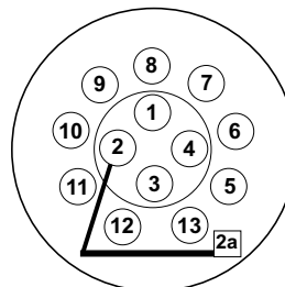
Johtojen liittäminen 13-napaiseen pistorasiaan
