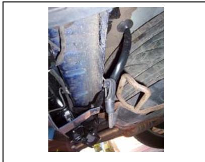
Kabelbaum AHK von Kabeldurchführung bis zur Steckdose verlegen
