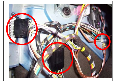
Anschluss E-Satz, Blinkerstecker links und Massekabel
