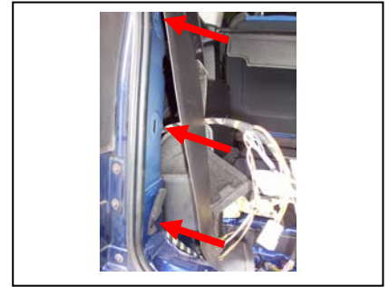
Linke Seitenverkleidung etwas abziehen, 3 Clips, Blinkerstecker verlegen
