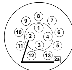
Připojení vodičů v 13-ti pólové zásuvce
